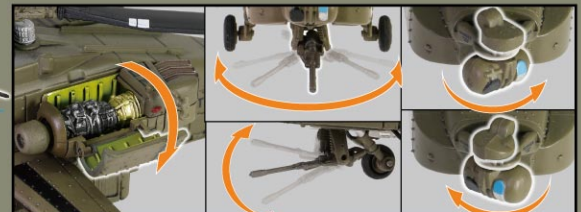
1)可打开的发动机舱门 2)M230链炮可转动和上下移动 3)夜视及红外前视仪可左右转动
